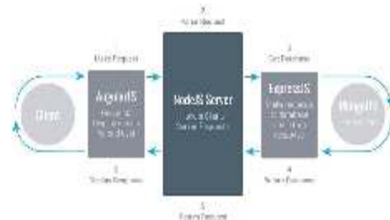
Gambar 6. Arsitektur PWA-MEAN
